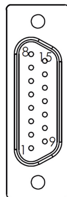
15针D型
