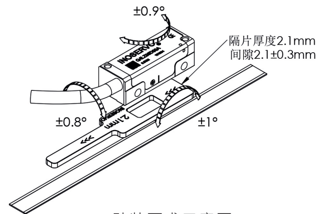
贴装要求示意图
