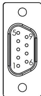
9针D型
