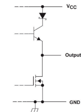
ABZ 信号输出电路图
